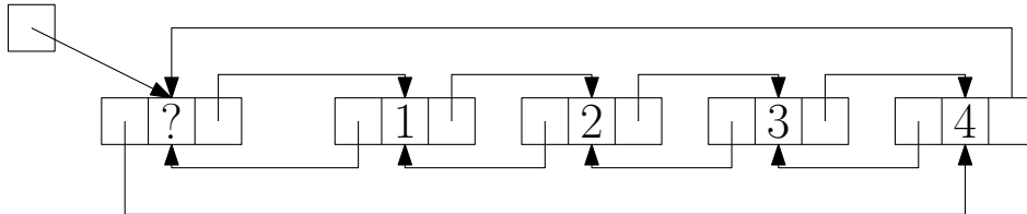
Liste doublement chaînée (1, 2, 3, 4), version avec sentinelle.
