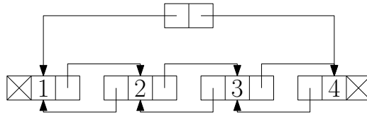
Liste doublement chaînée (1, 2, 3, 4), première version.
